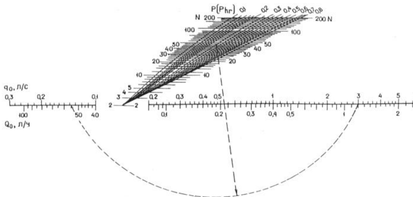
Черт. 3. Номограмма для определения секундных и часовых расходов воды q при q_0 \leq 0,3 л/с, N \leq 200 и P > 0,1
